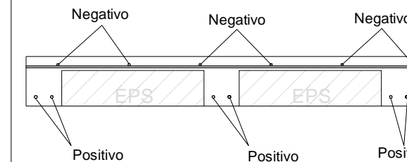
LAJE NERVURADA
