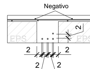
DET. ARMADURA POSITIVA
